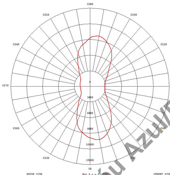
Figura 5 - Curva de intensidade máxima para cada ângulo C (51239-2).
