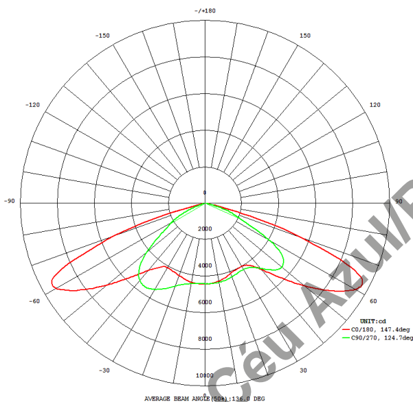
Figura 1 - Curva de distribuição de intensidade luminosa (51239-1).
